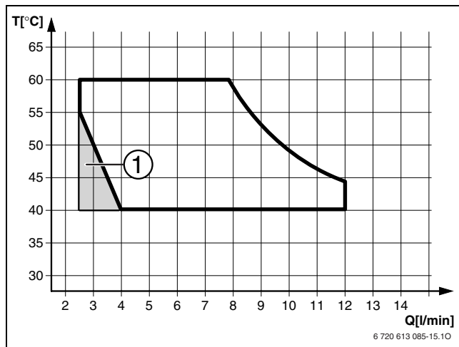
10. ábra +15°C befolyó hidegvíz hőmérséklet diagramm (ZWE 24-5 MFA/MFK)
