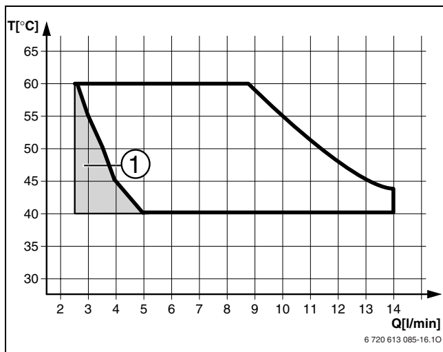
11. ábra +15 °C befolyó hidegvíz hőmérséklet diagramm (ZWE 28-5 MFA)
